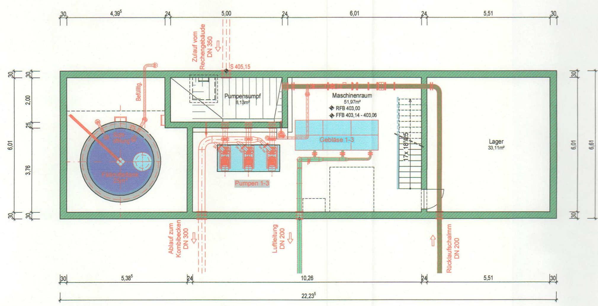
Grundriss Kellergeschoss
