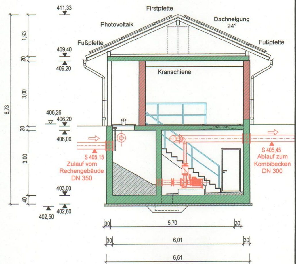
Schnitt C - C
