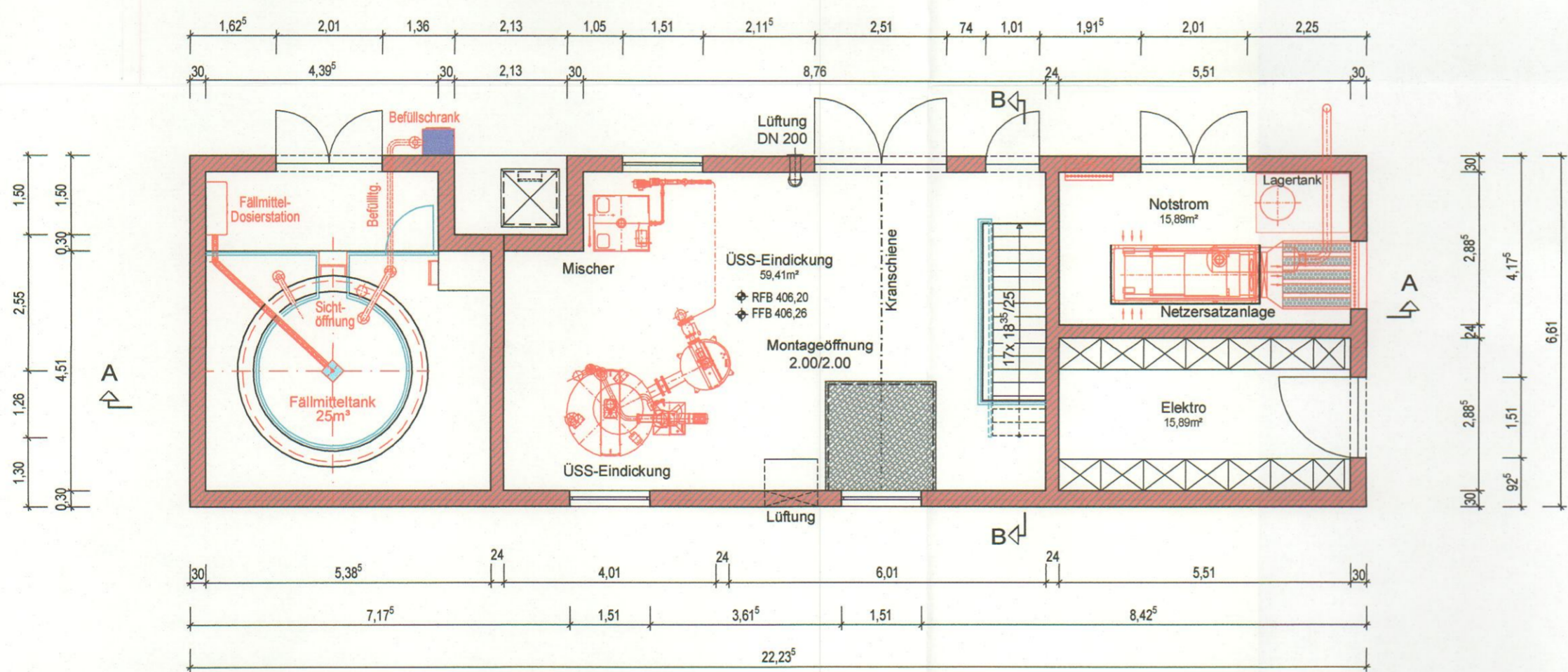
Grundriss Erdgeschoss
