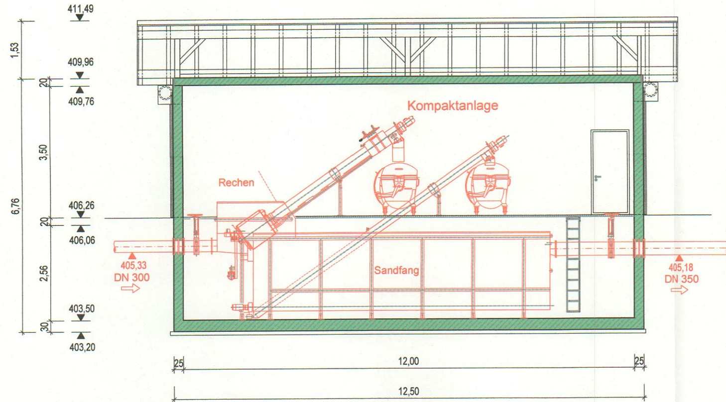
Schnitt A - A
